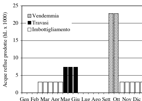
Figura 5.2. Stima dei volumi di acque reflue prodotte in una cantina in funzione delle diverse operazioni di lavorazione.
