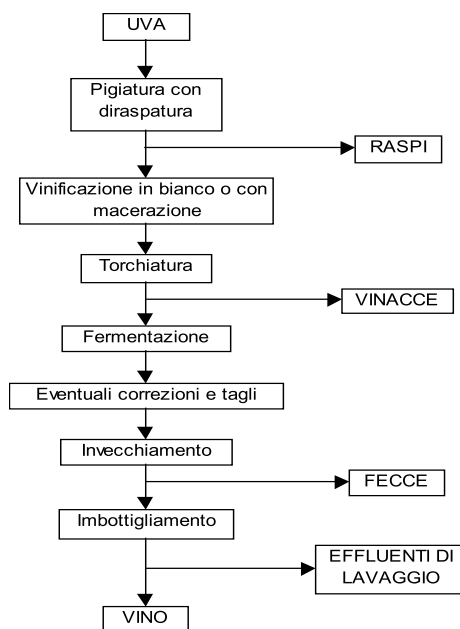
Figura 5.1. Schema sintetico del processo di produzione del vino.
